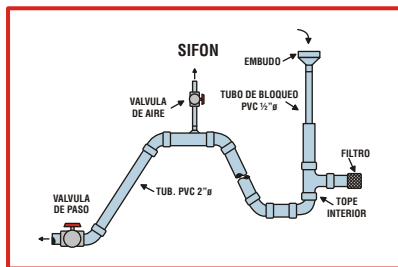
Figura N° 5: Esquema del diseño del sifón
