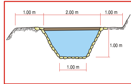
Figura N° 2: Sección del Reservorio
